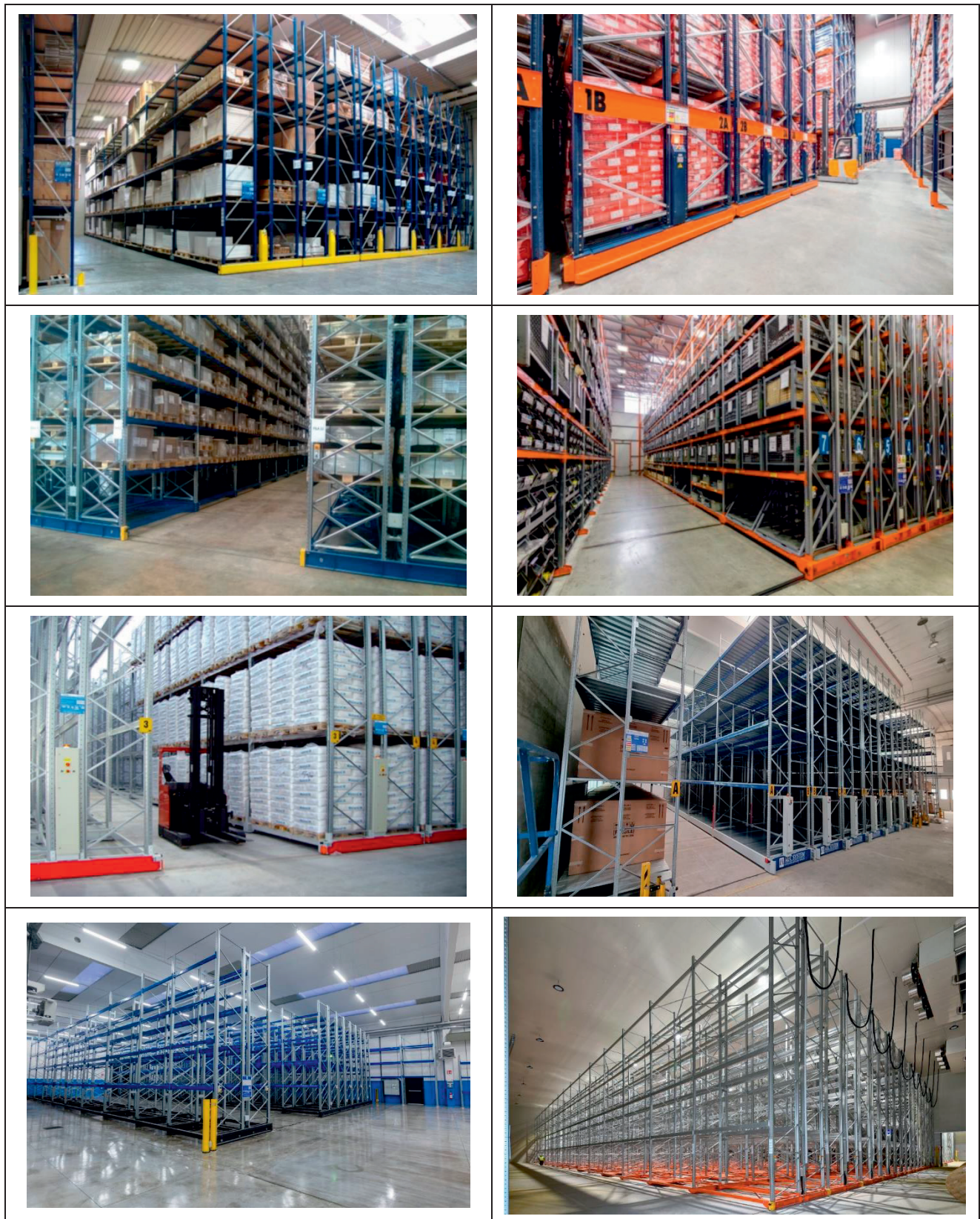
Figura B-4: Scaffalature mobili - classificazione 5.5.1 UNI EN 15878
