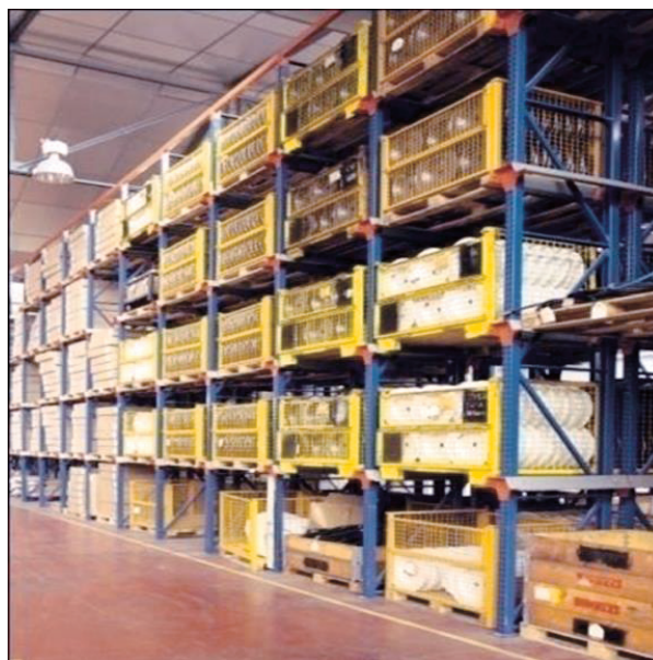
Figura 1-3: Scaffalatura porta pallet a fronte libero
