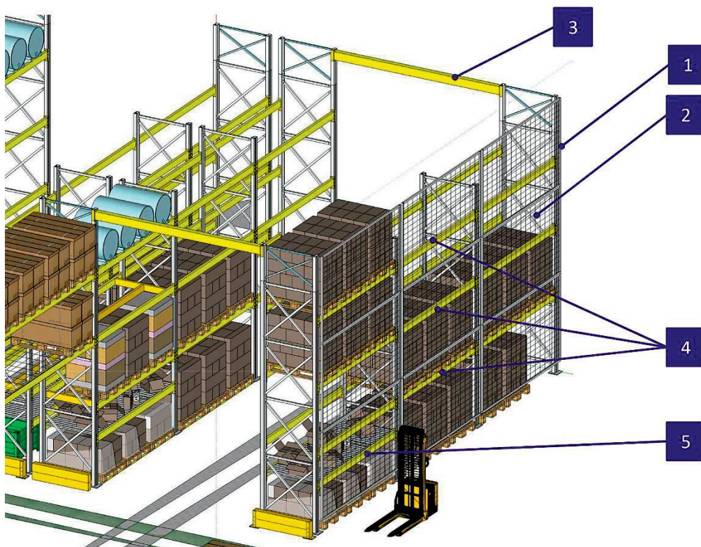
Figura A-6: Scaffalatura vista dal corridoio di servizio
