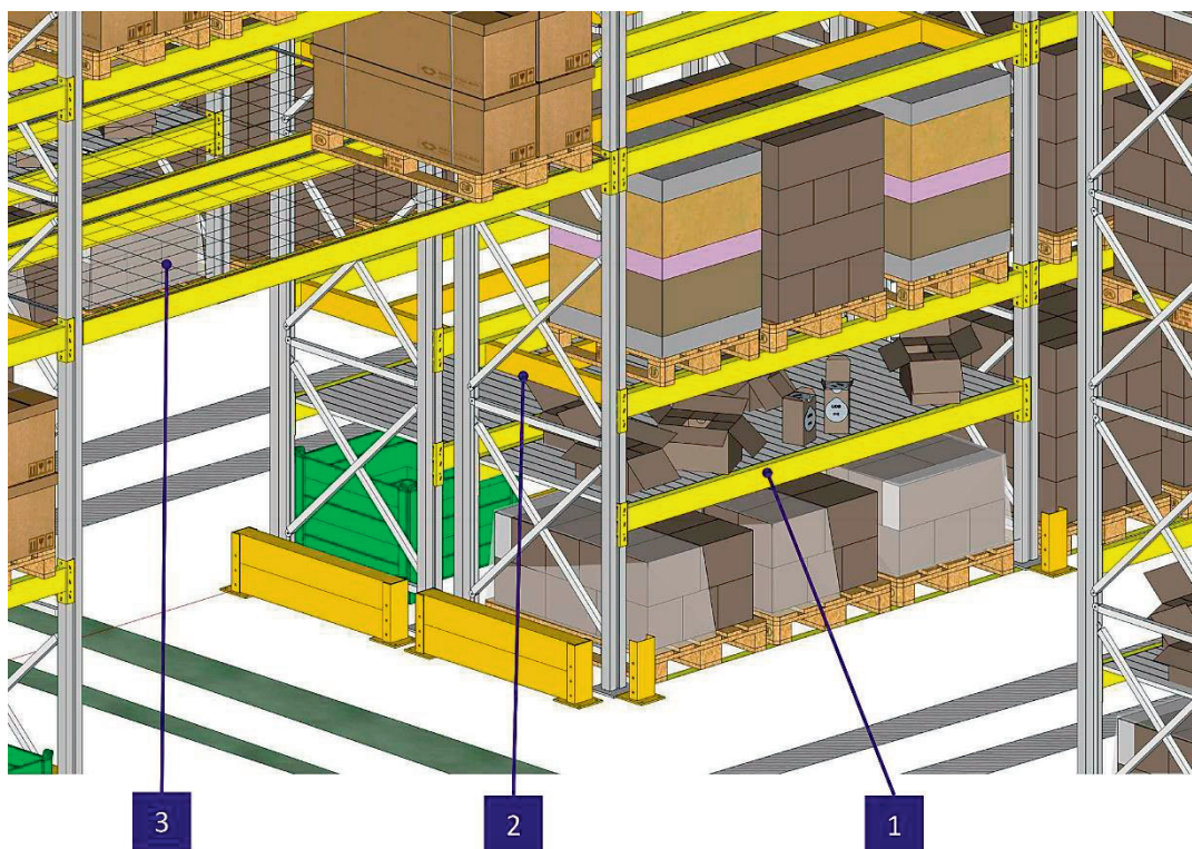
Figura A-5: Scaffalatura accessoriata
